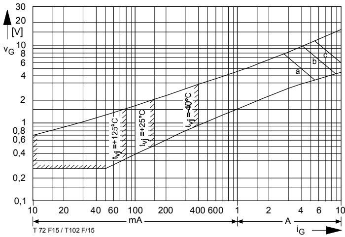
Bild / Fig. 15 Zündbereich und Spitzensteuerleistung bei v_D = 6 \text{ V} . Gate characteristic and peak power dissipation at v_D = 6 \text{ V} . Parameter: a b c
